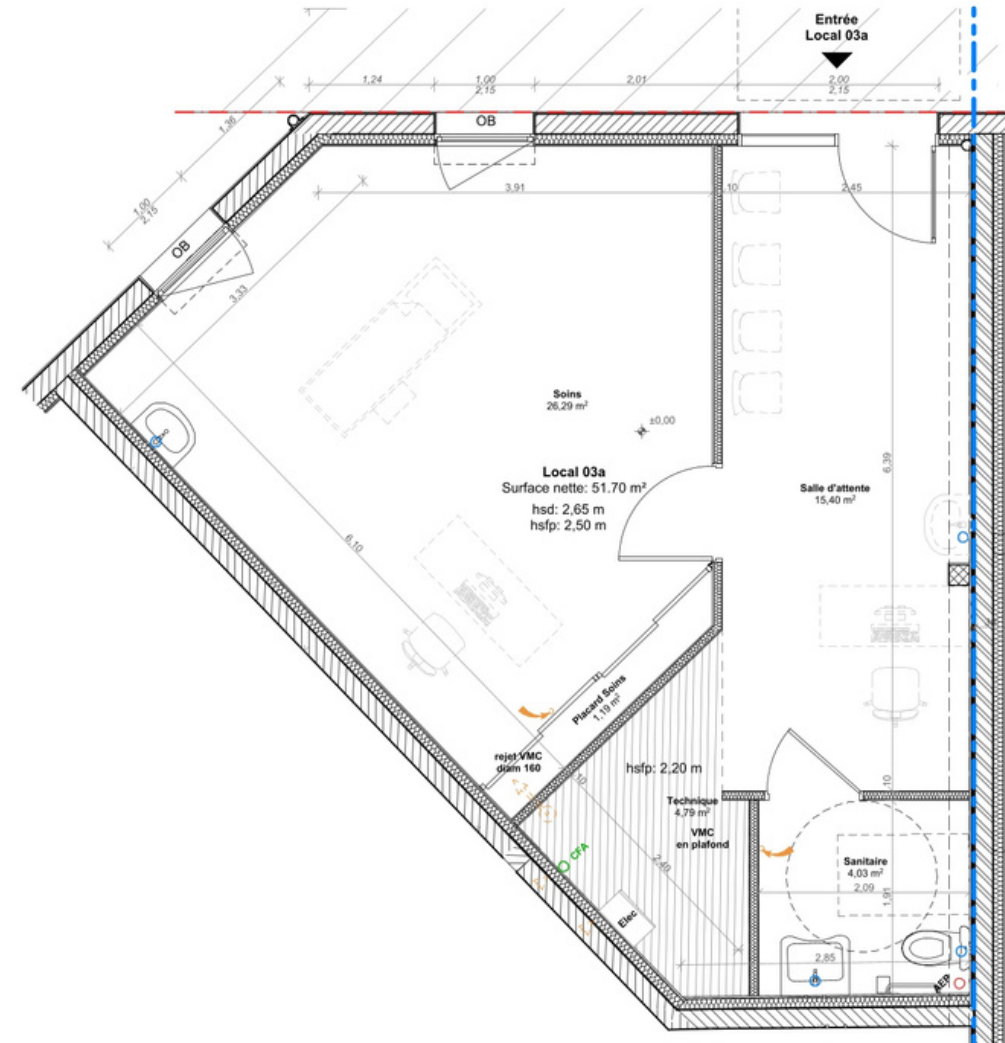
Plan du Rez-de-chausée
