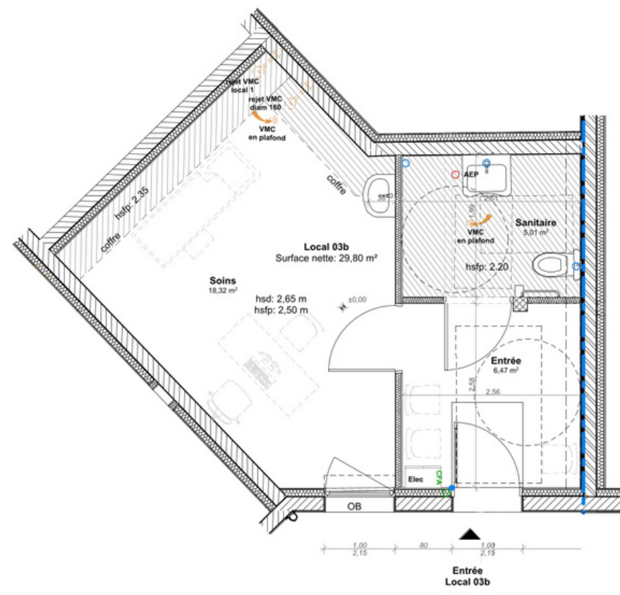
Plan du Rez-de-chausée
